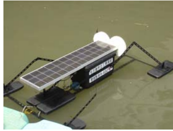
480 エコむし1 水中に空気を送り込んで堀川を きれいにする浄化ロボット
